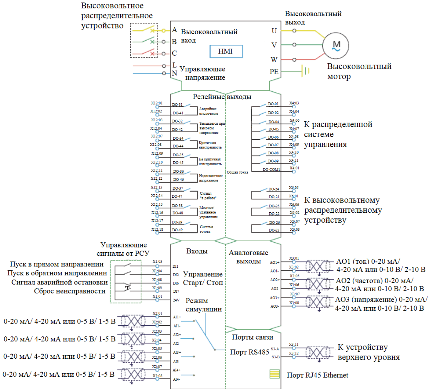
Рисунок 12 – Схема внешних подключений ПЧ ES9000
