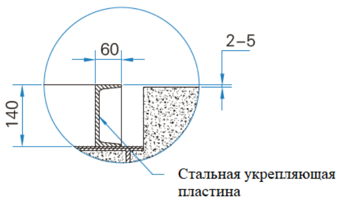
Рисунок 12 – Схема фундамента для монтажа
