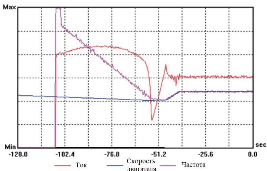
Рисунок 11 – Диаграмма перезапуска с отслеживанием скорости
