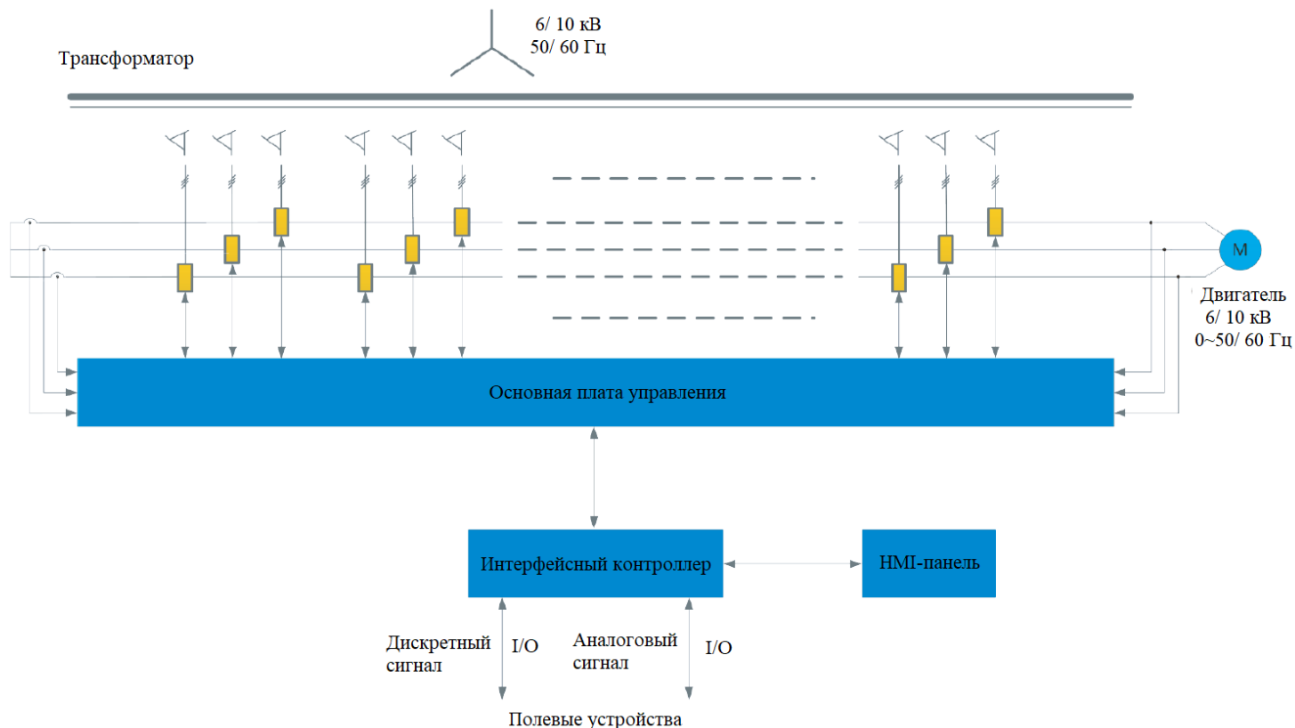
Рисунок 9 – Функциональная схема преобразователя частоты
