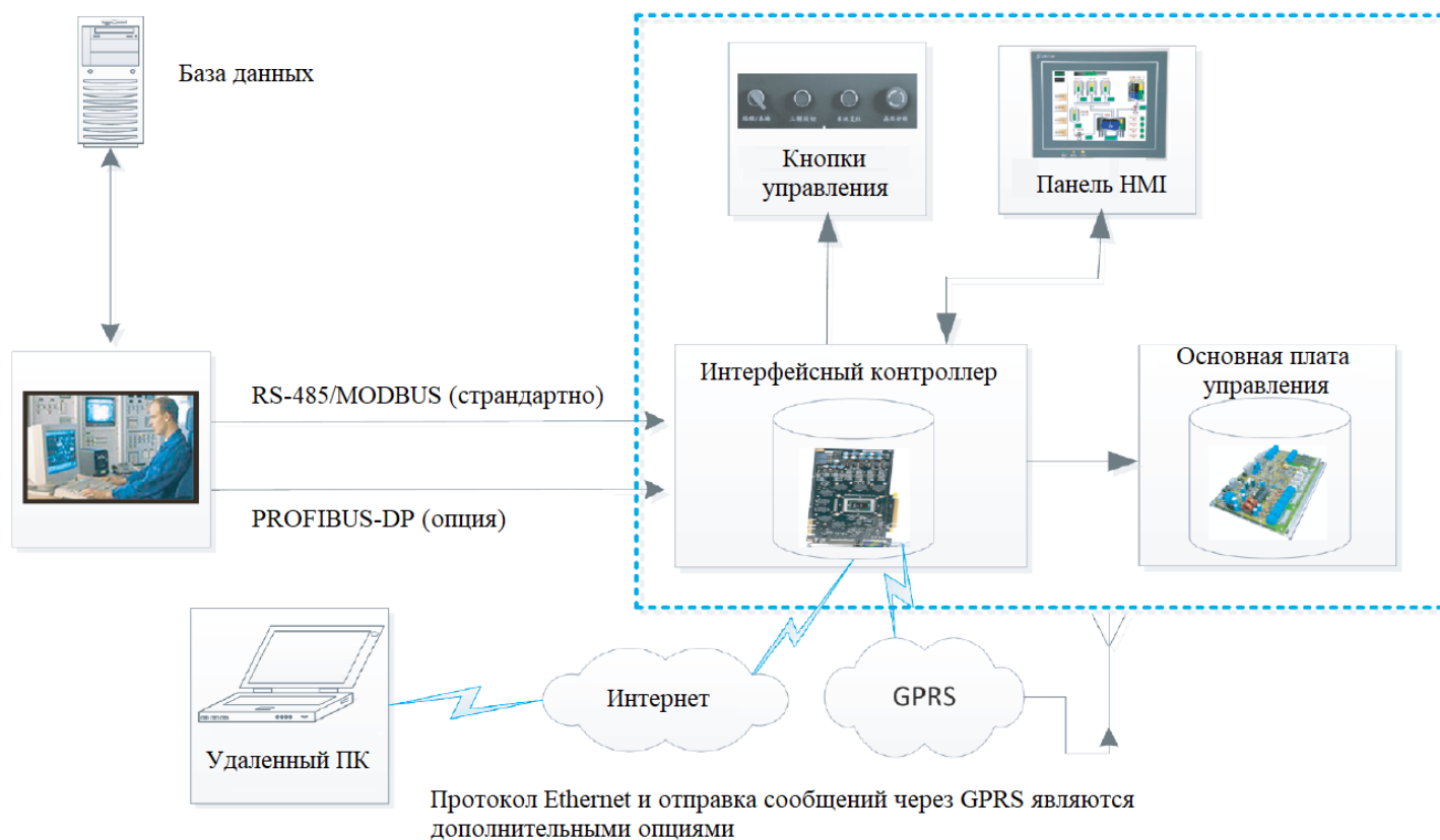
Рисунок 10 – Организация системы управления и связи
