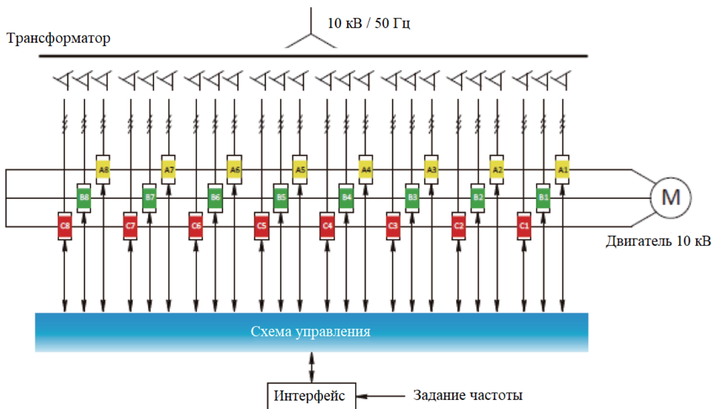
Рисунок 5 – Блок-схема ПЧ ES9000 с выходным напряжением 10 кВ
