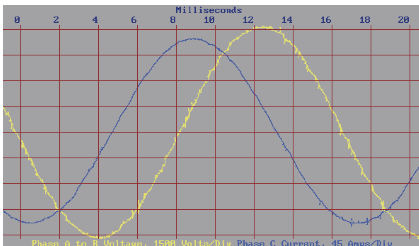
Рисунок 6 – Форма выходного напряжения и тока
