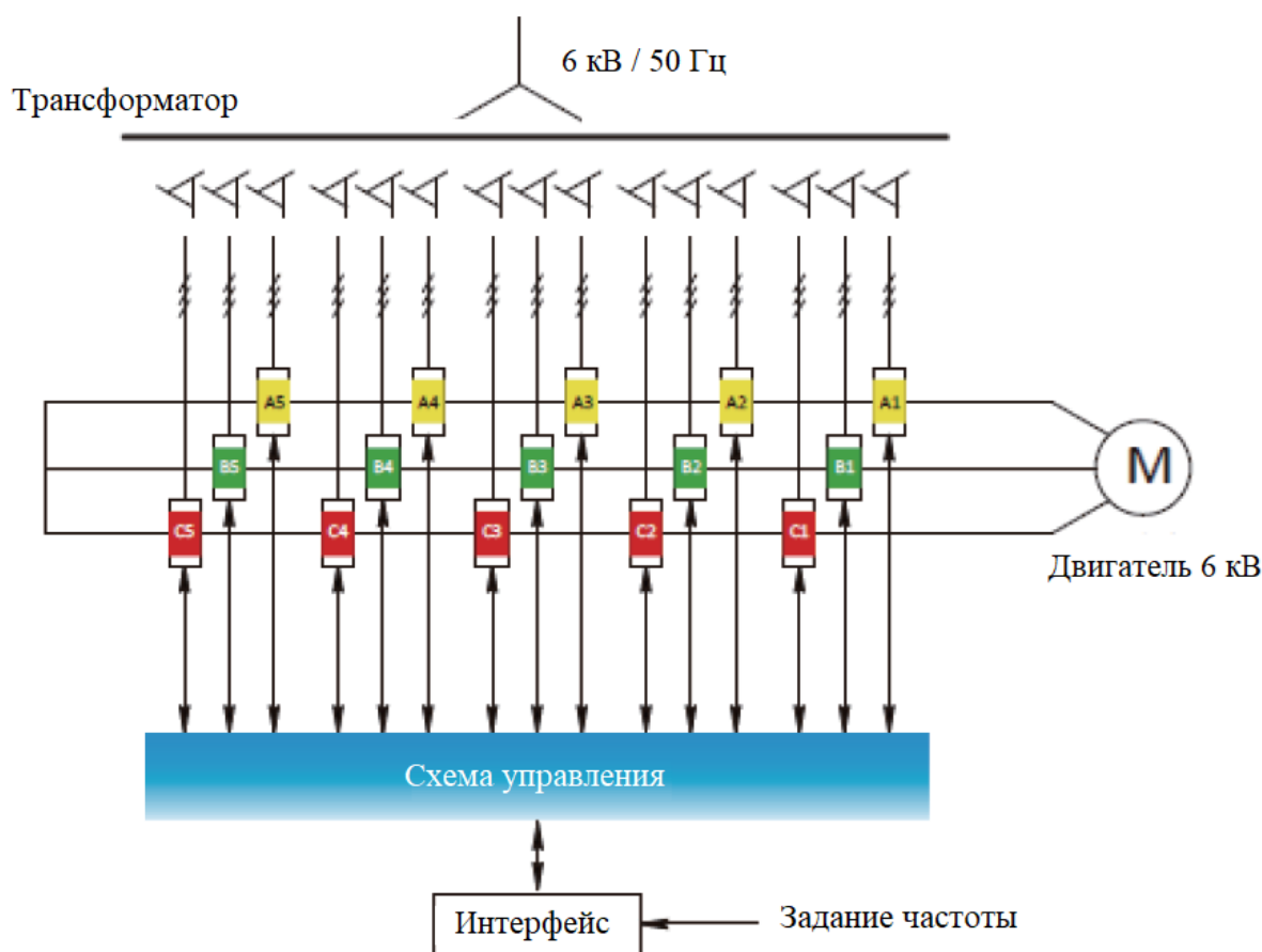
Рисунок 4 – Блок-схема ПЧ ES9000 с выходным напряжением 6 кВ
