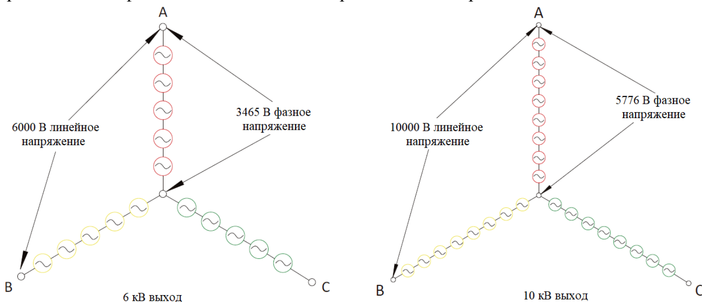
Рисунок 7 - Схема суммирования напряжений для ПЧ с силовыми ячейками в фазе
