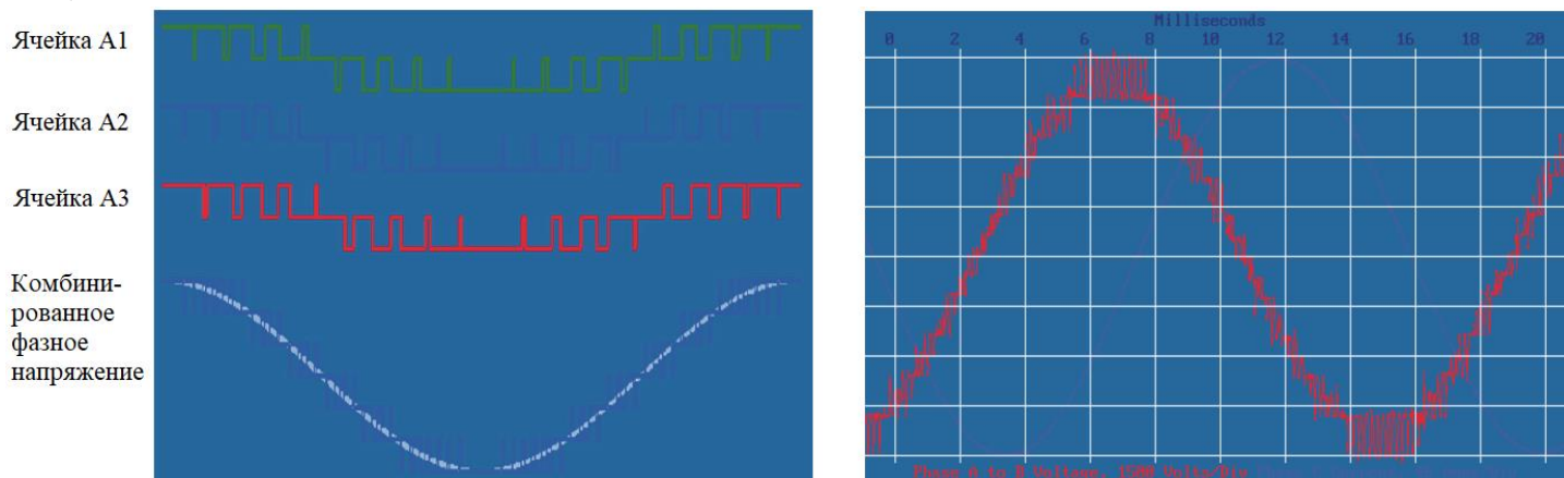
Рисунок 8 – Сложение сигналов ячеек и фактическое линейное напряжение
