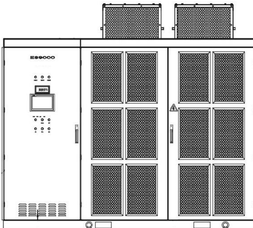
Рисунок 1 – Преобразователь частоты ES9000 интегрированного исполнения
