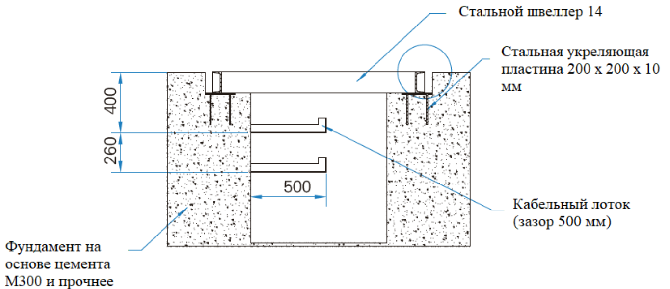
Рисунок 14 – Схема фундамента для монтажа
