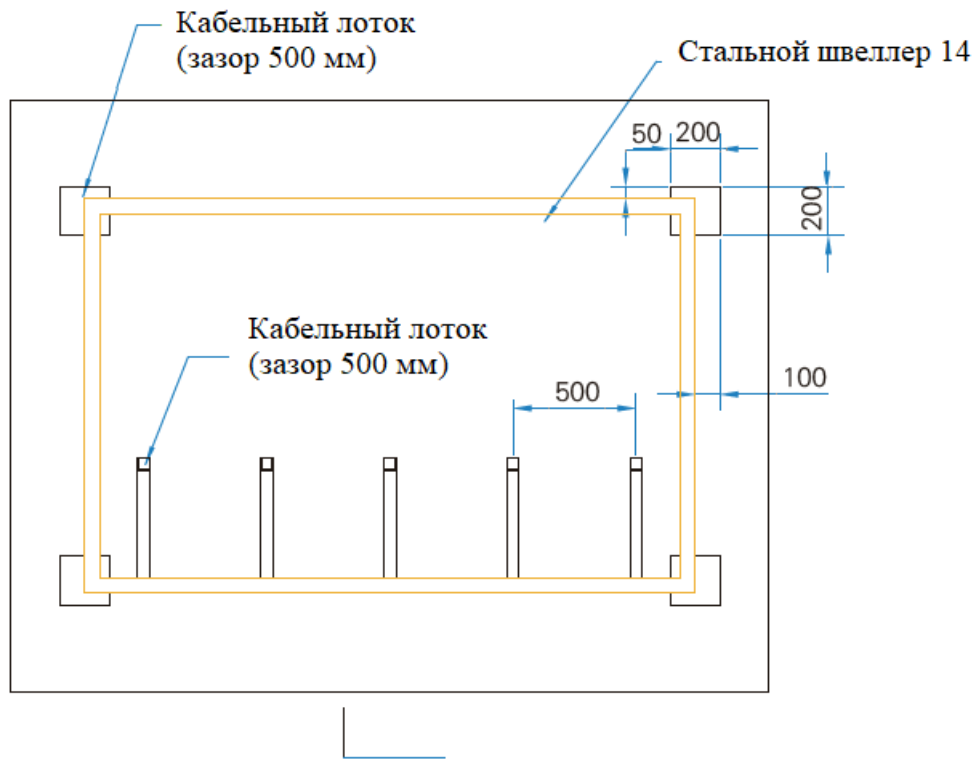
Рисунок 13 – Схема фундамента для монтажа
