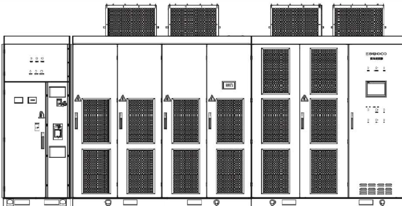
Рисунок 2 – Преобразователь частоты ES9000 секционного исполнения
